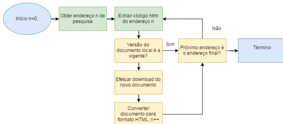
FIGURA 1 – Fluxograma básico do MPObot
